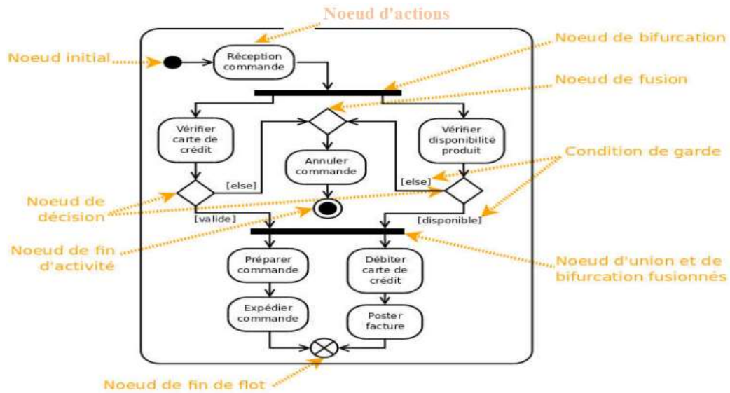
Exemple de diagramme d'activité
